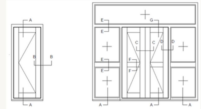
FLUSH DOOR SD OUT - FRAME OVOLO/ SQUARE
