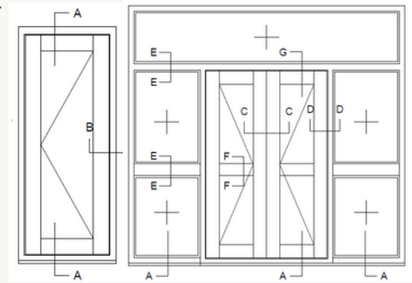
FLUSH DOOR OUT
