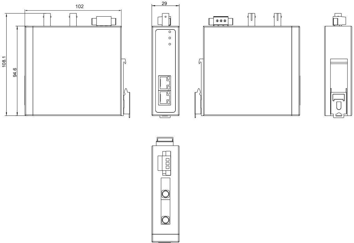
DSW-ECT-A4K0202-S-STA DSW-ECT-A4K0202-S-STB
