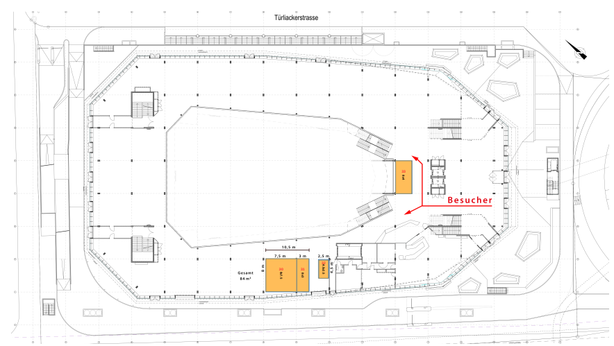
Hallenplan Erdgeschoss
